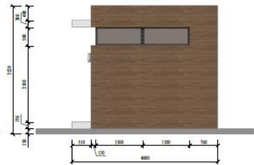
ФАСАД 4
