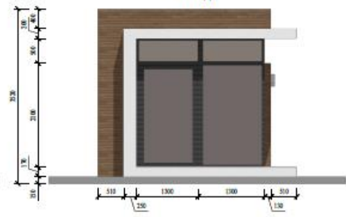
ФАСАД 4
