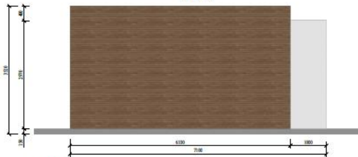
ФАСАД 3
