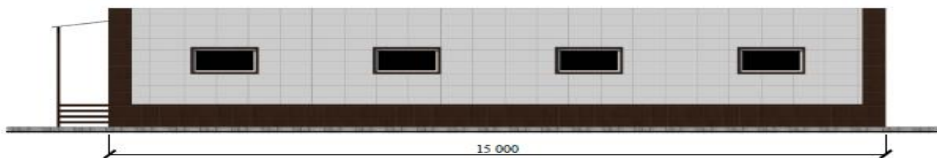
ФАСАД 2
